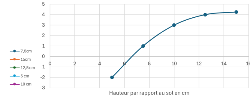
Angle Cl max en fonction de la hauteur par rapport au sol
